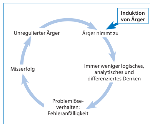
Abbildung 9 Problemlösedynamik bei Black Jack
